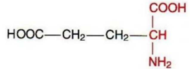
Acide glutamique (Glu, E)
