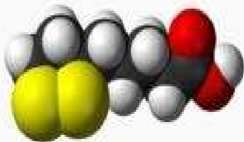
Structure de l'acide lipoïque
