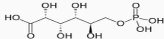
Structure de l'acide 6-phosphogluconique
