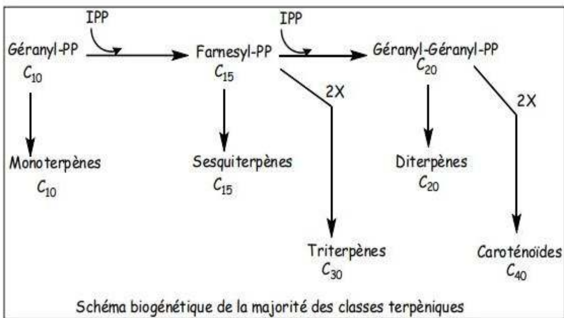
Figure 2 : Polymérisation successive d'IPP- conversion en terpénoïdes supérieurs.
